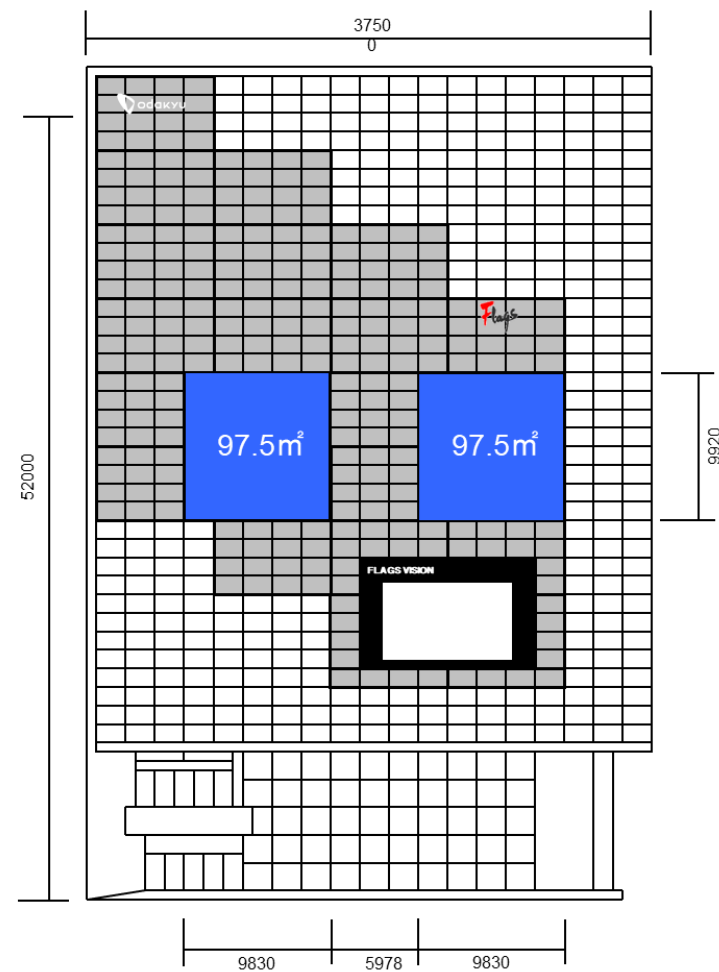
立面図（2面）
