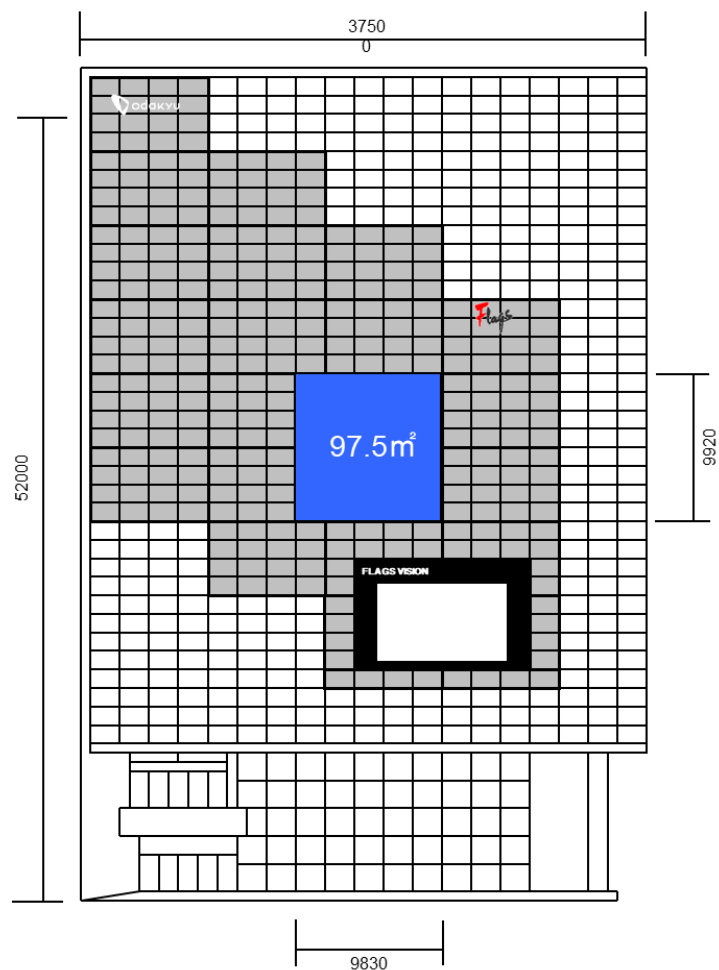
立面図（1面）
