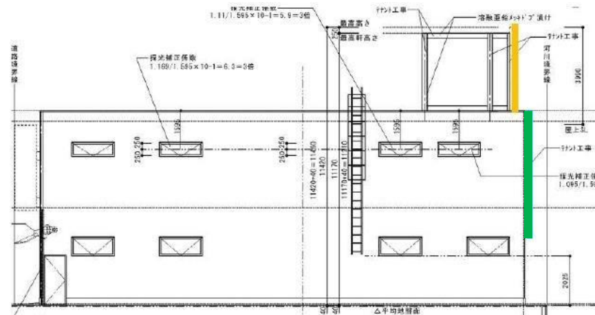
断面図
