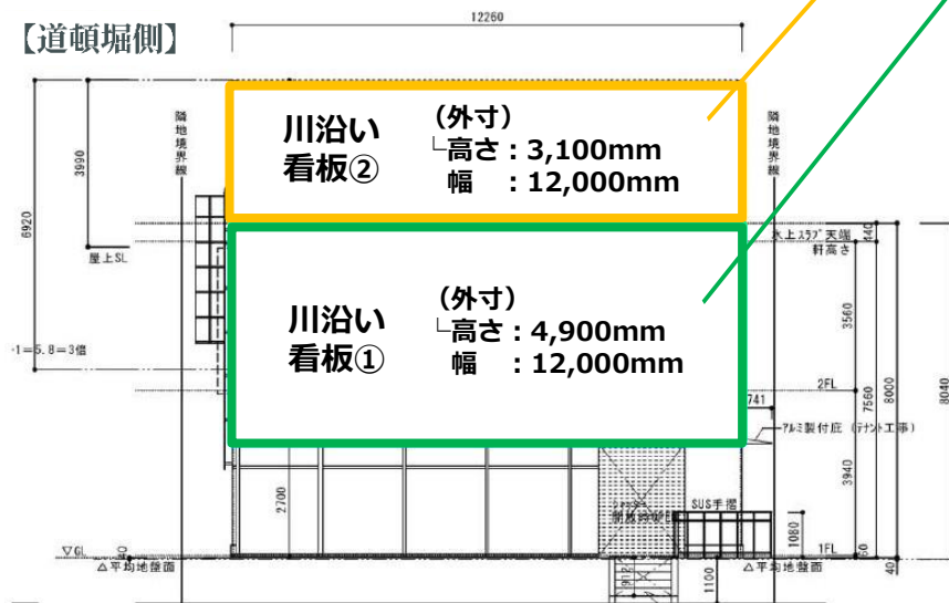
立面図
