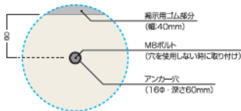
部分拡大図B(正面図)
