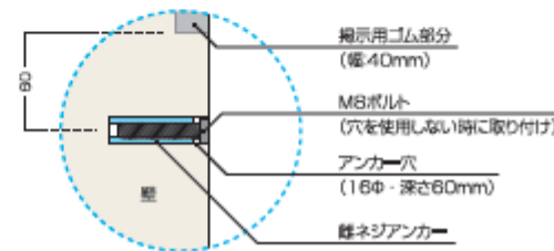
部分拡大図B(断面図)
